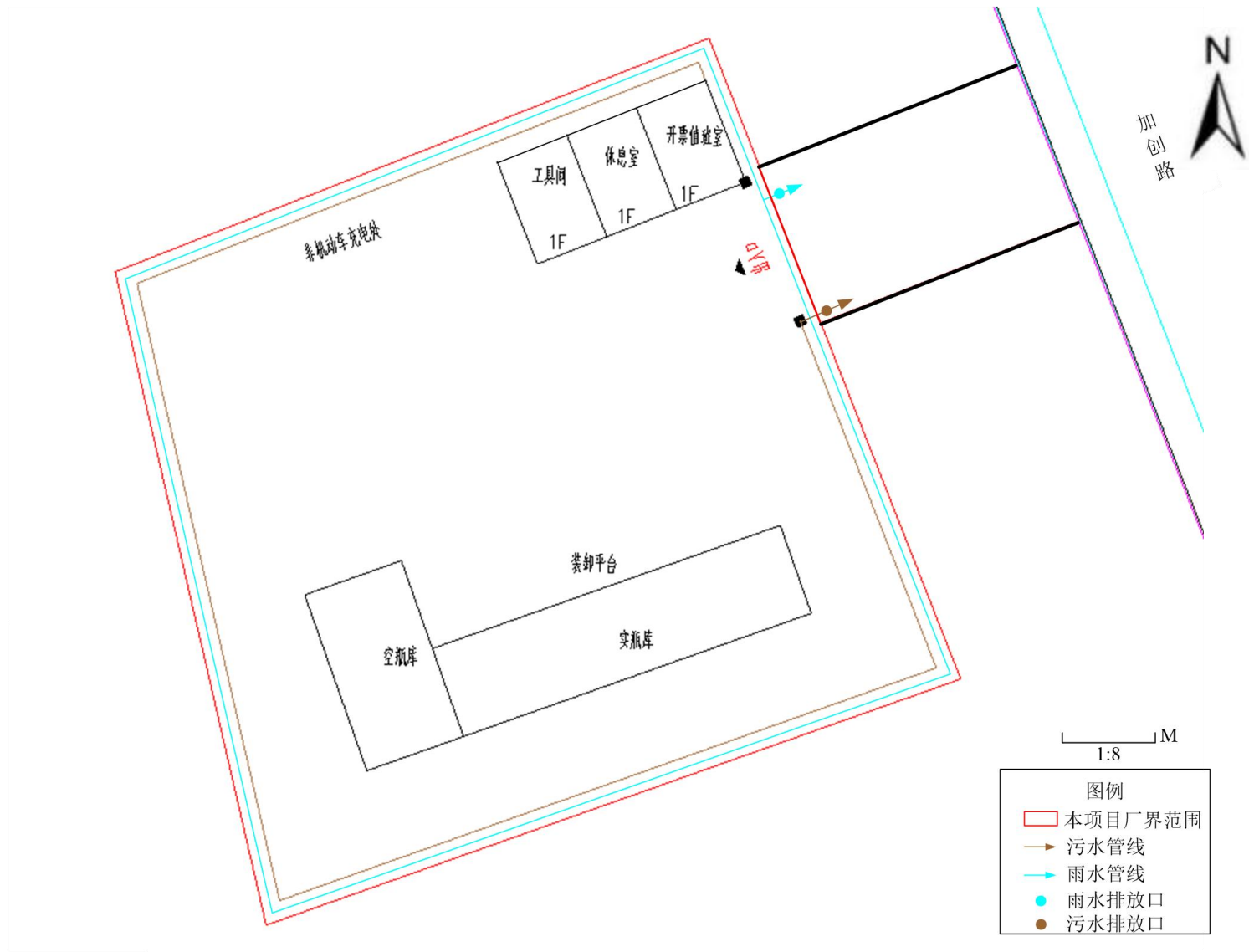
附图 5 厂区平面布置图
