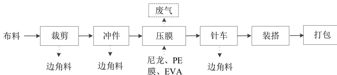
图 2 布箱包工艺流程图
