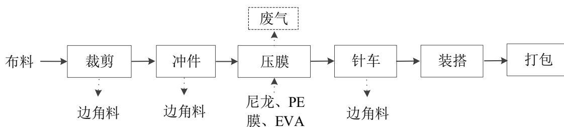
图 2.2.1-2 布箱包工艺流程图
